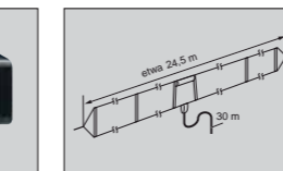
AH-710 DIPOL-ANTENNE Frequenzbereich 1,9 bis 30 MHz. PL-259-Anschluss. Einfach zu montieren (ausgereifte Konstruktion).
